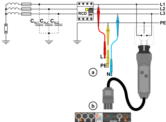
Rys. 3.7 Pomiar RCD w sieci IT. Obwód zamyka się przez pojemności pasozytne C_x
